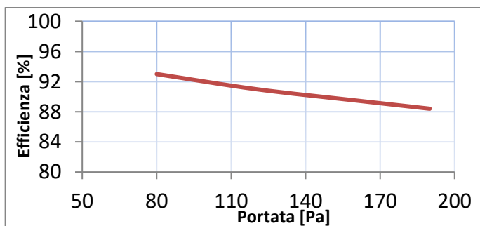
Curva di prestazione RCE 016
