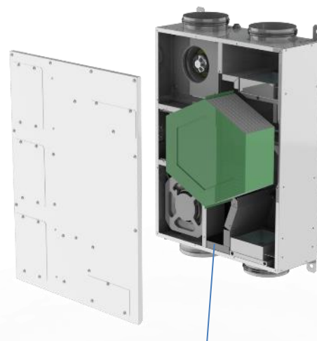
VASCHETTA DI RACCOLTA CONDENSA
