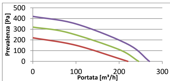
Curva portata – prevalenza RCE 022
