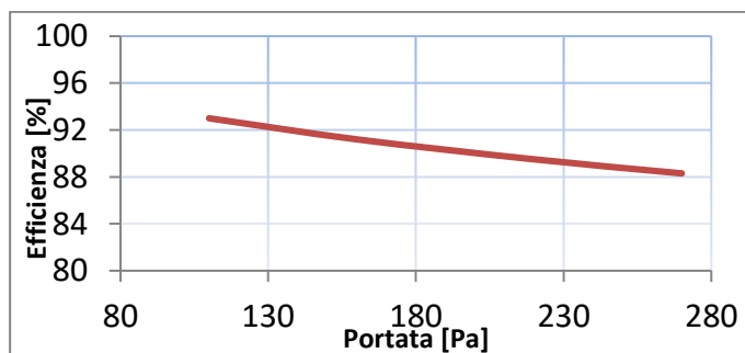
Curva di prestazione RCE 022
