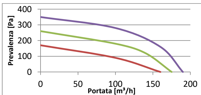
Curva portata – prevalenza RCE 016
