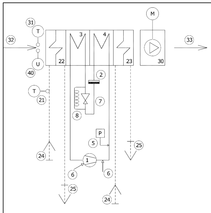
Modello 050_A (isotermico)
