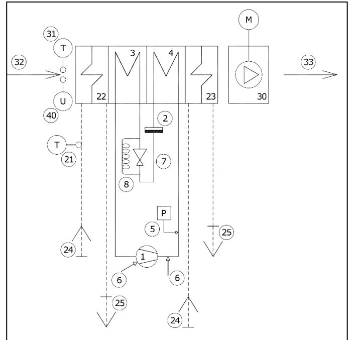
Modelli 050_070_A (isotermico)
