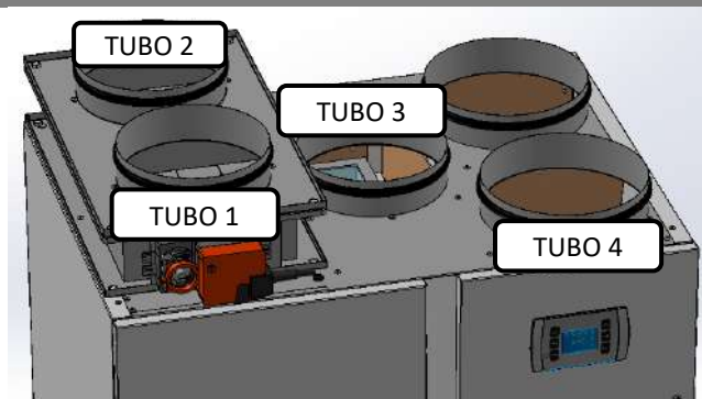
REV 050 e REV 070 VISTA IN ALTO
