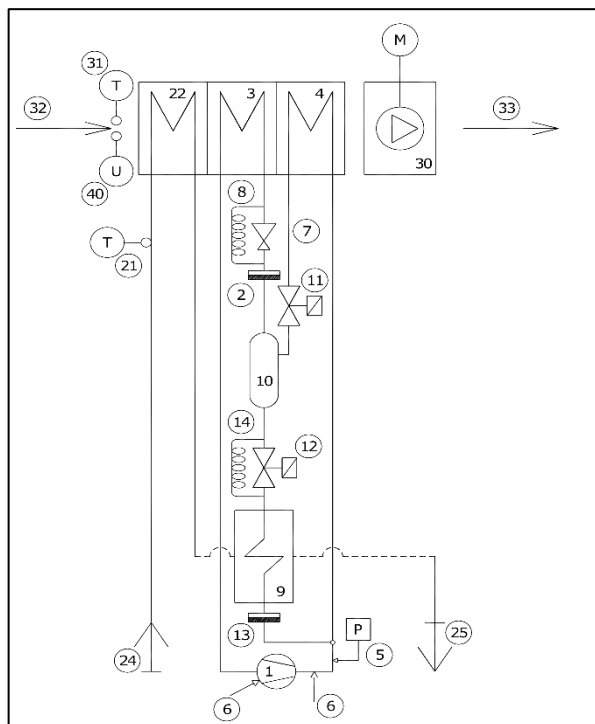
RS_100_I (ibrido)
