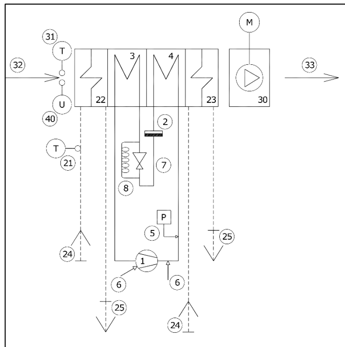
RS_050_A (isotermico)
