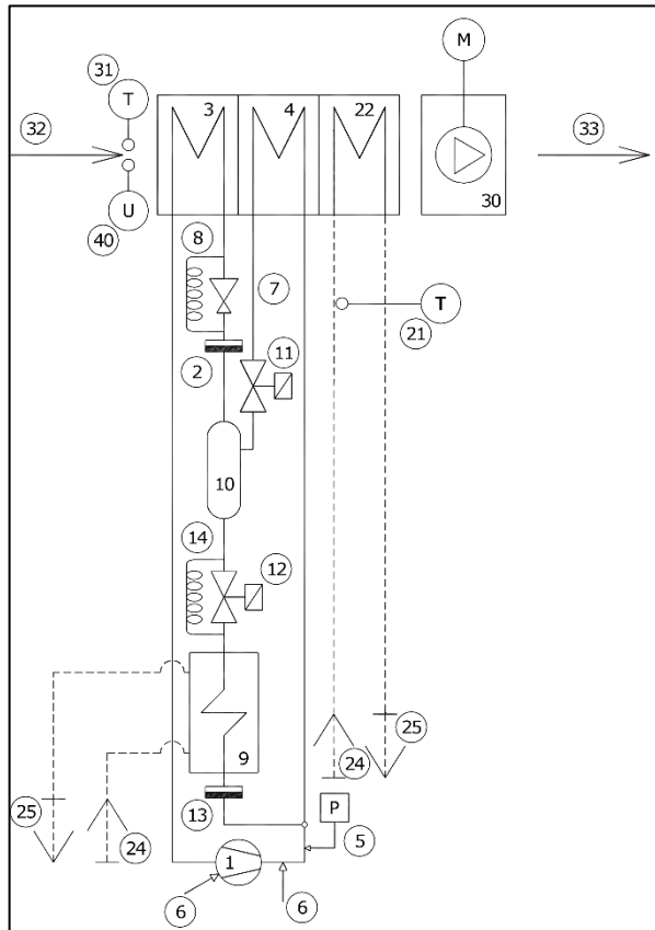
RS_100_I (ibrido)
