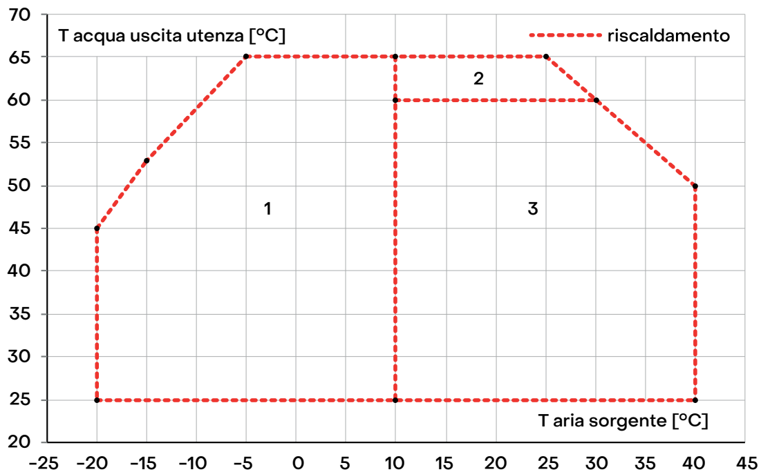
» Limiti di funzionamento NAW in riscaldamento per acqua prodotta e temperatura aria esterna (taglie 006-017)
