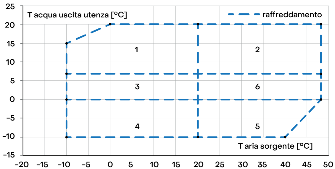
» Limiti di funzionamento NAW in raffreddamento per acqua prodotta e temperatura aria esterna (taglie 006-017)
