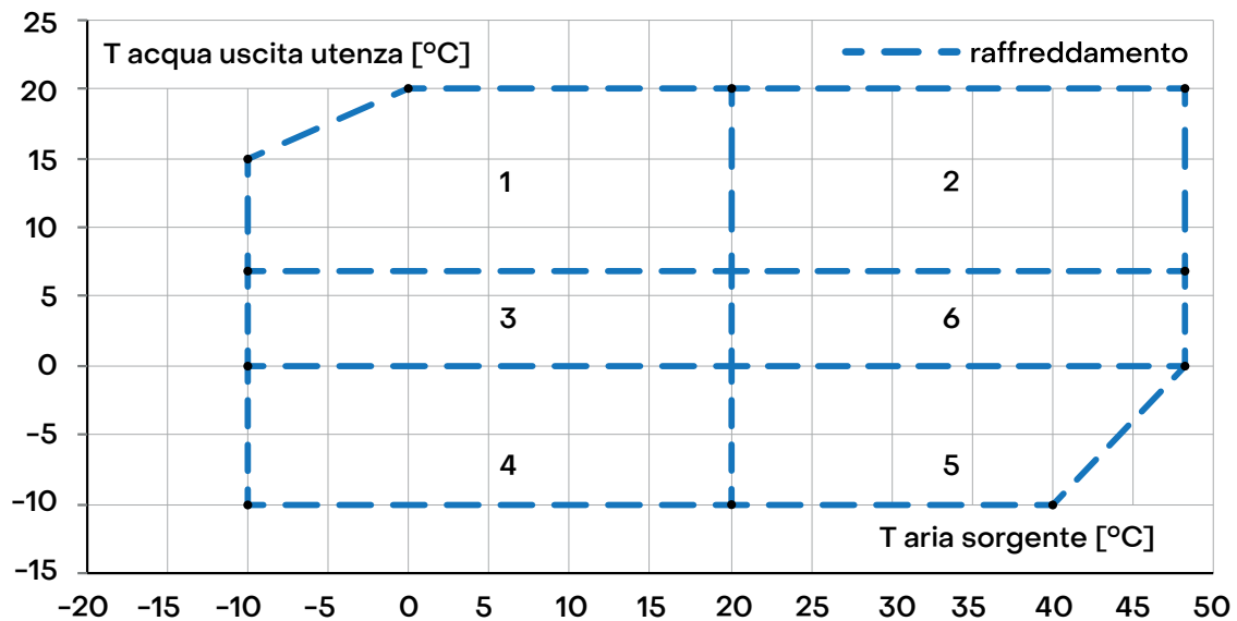
» Limiti di funzionamento RAW in raffreddamento per acqua prodotta e temperatura aria esterna
